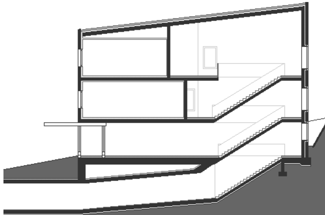
Schnitt
